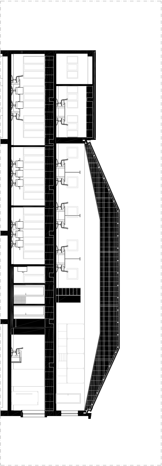
0 1 2 3 4 5 Corte AB
