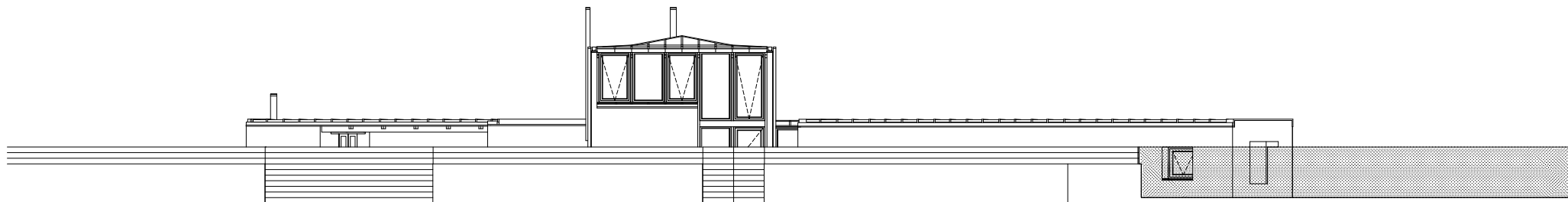
ALÇADO NORDESTE COM MURO
