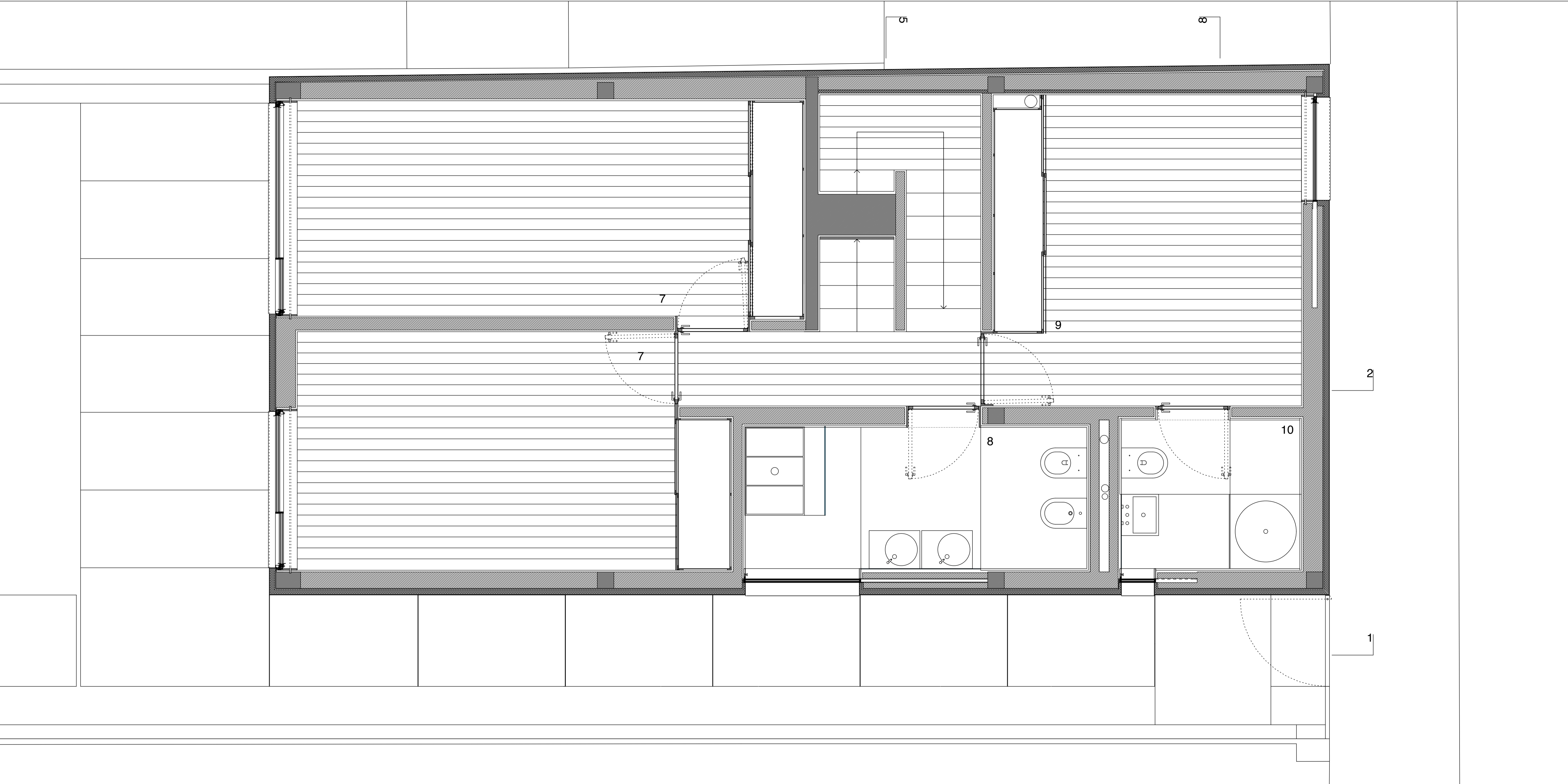
planta piso 1 | 7_Quartos 8_I.S. de apoio aos quartos 9_Quarto Suit 10_I.S. de apoio a suit
