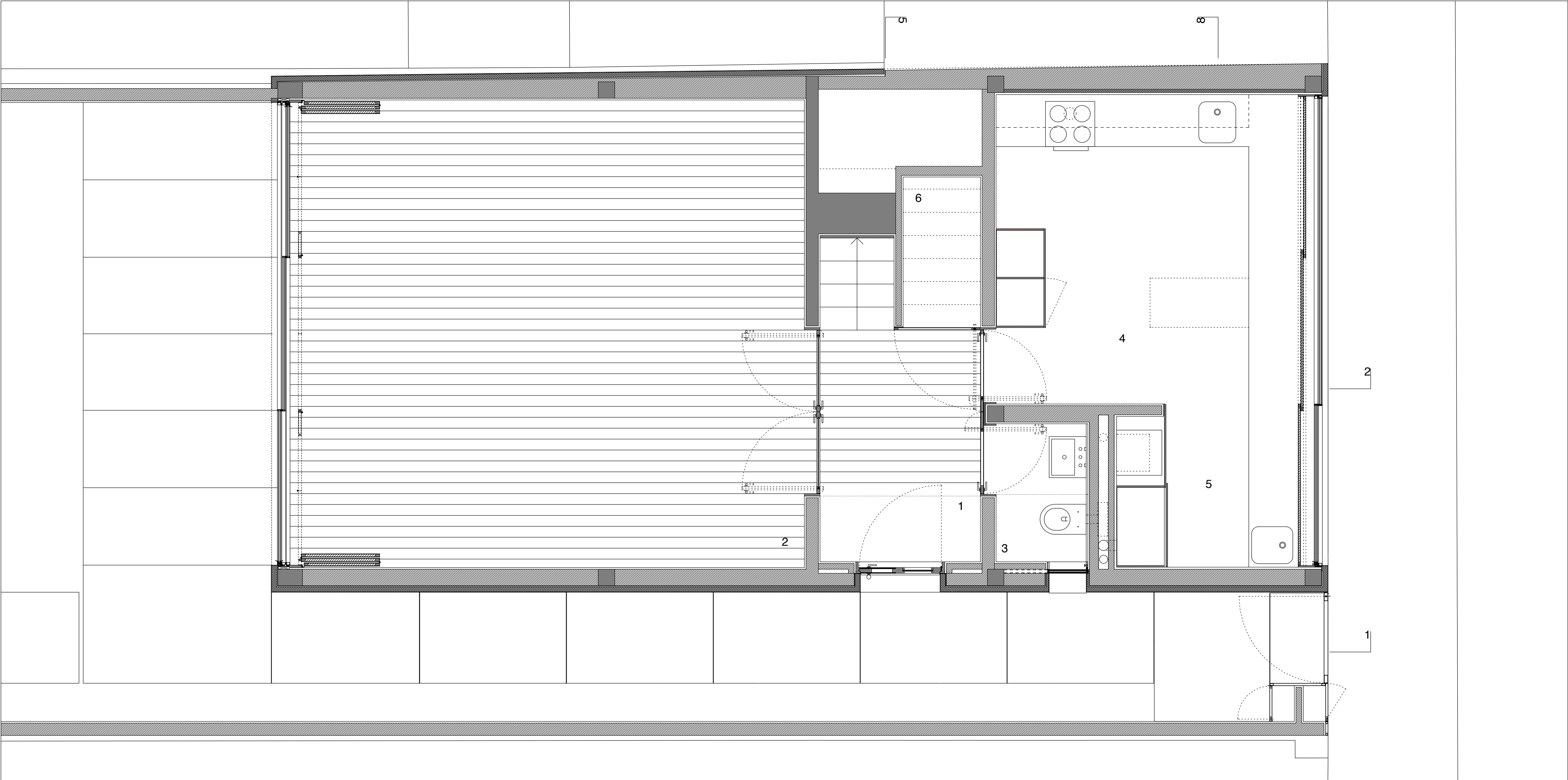
planta piso 0 | 1_Entrada 2_Sala 3_I.S. Serviço 4_Cozinha 5_Lavandaria 6_Despensa
