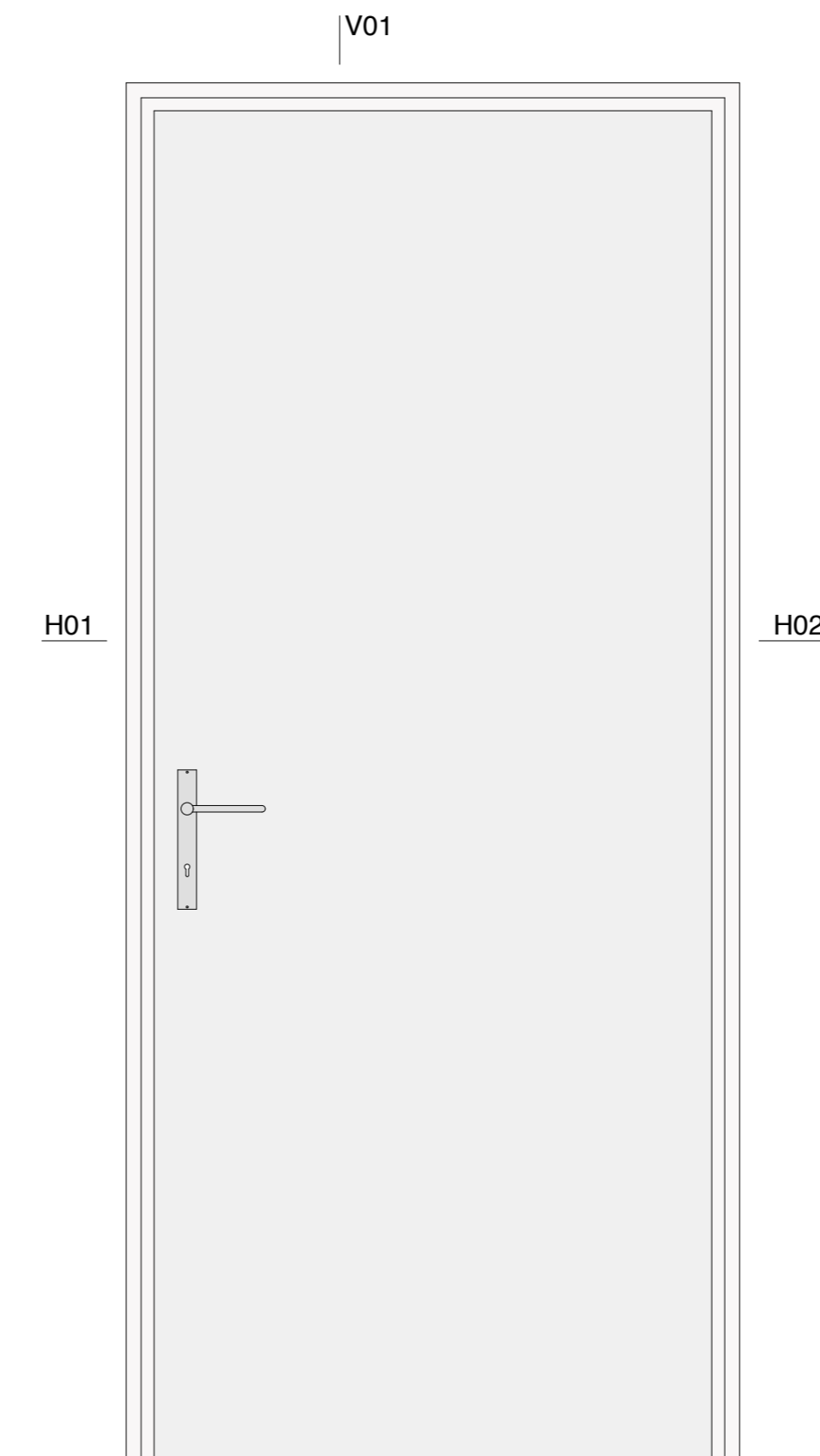
Alçado exterior - Porta tipo
