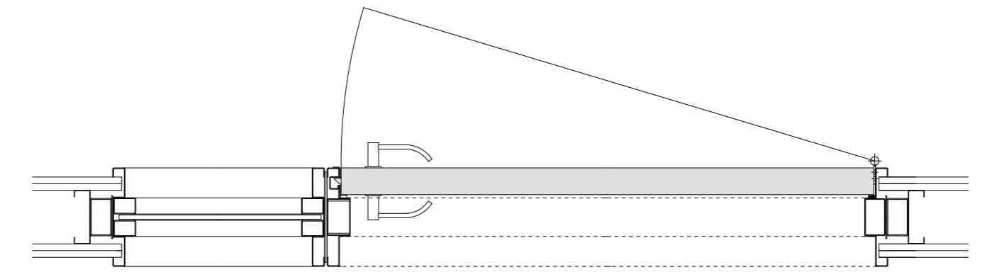
Planta - Porta tipo da sala de aulas
