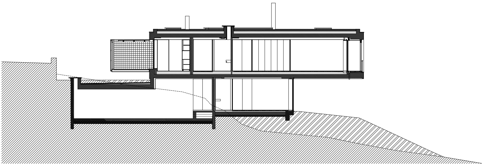
CORTE C2
