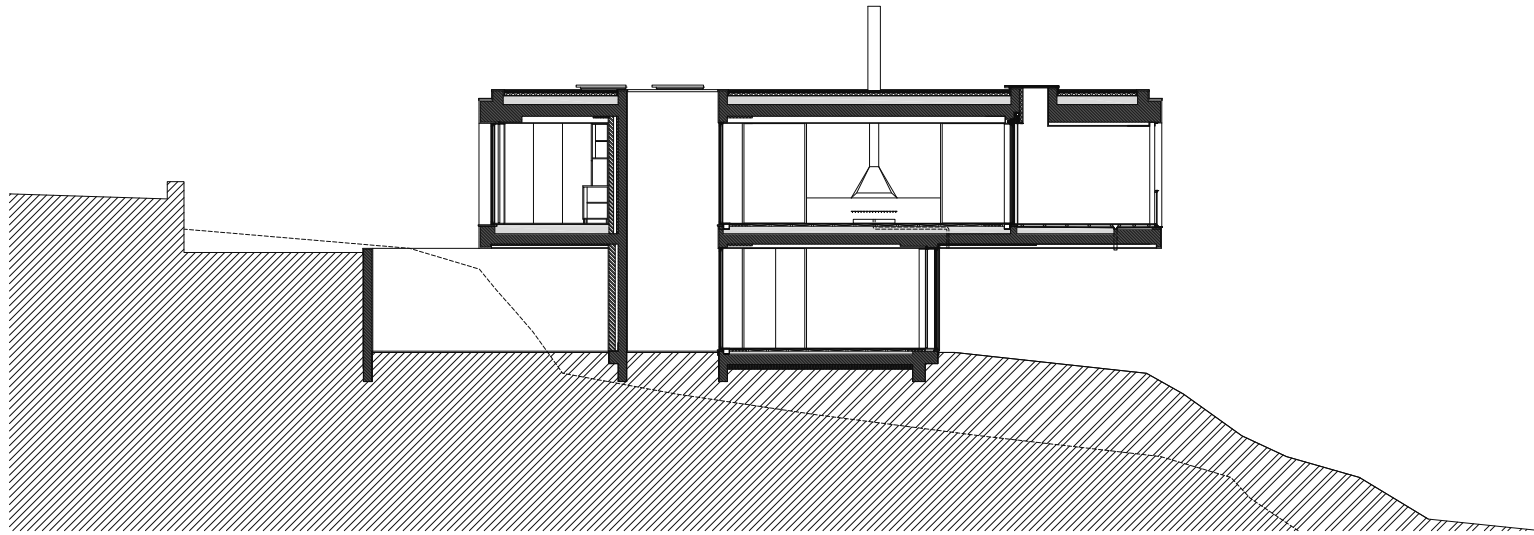
CORTE C1
