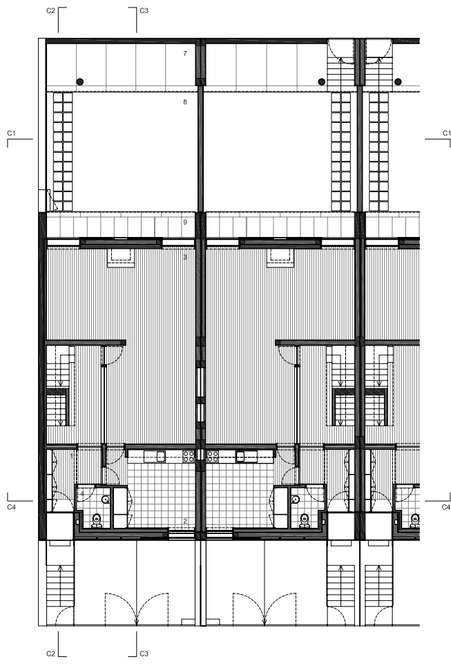
planta piso 1
