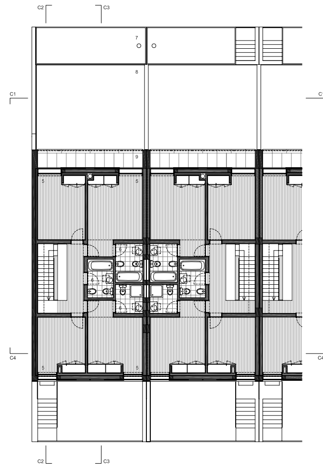
planta piso 2
