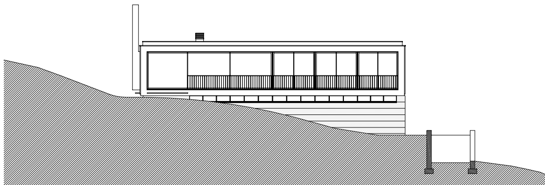
alçado sul
