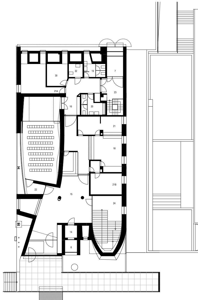
0 2 5 10m PLANTA PISO 0
