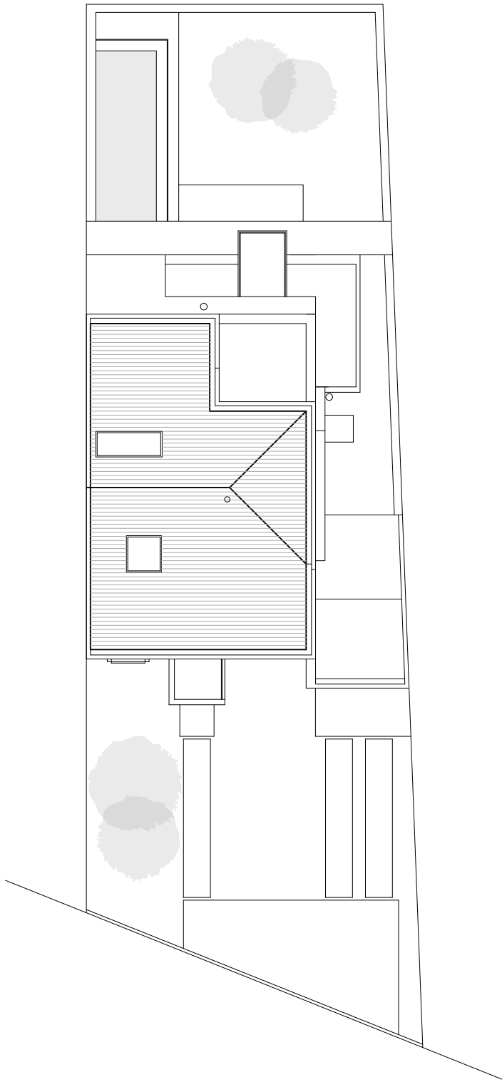
0 1 2 5m PLANTA COBERTURA
