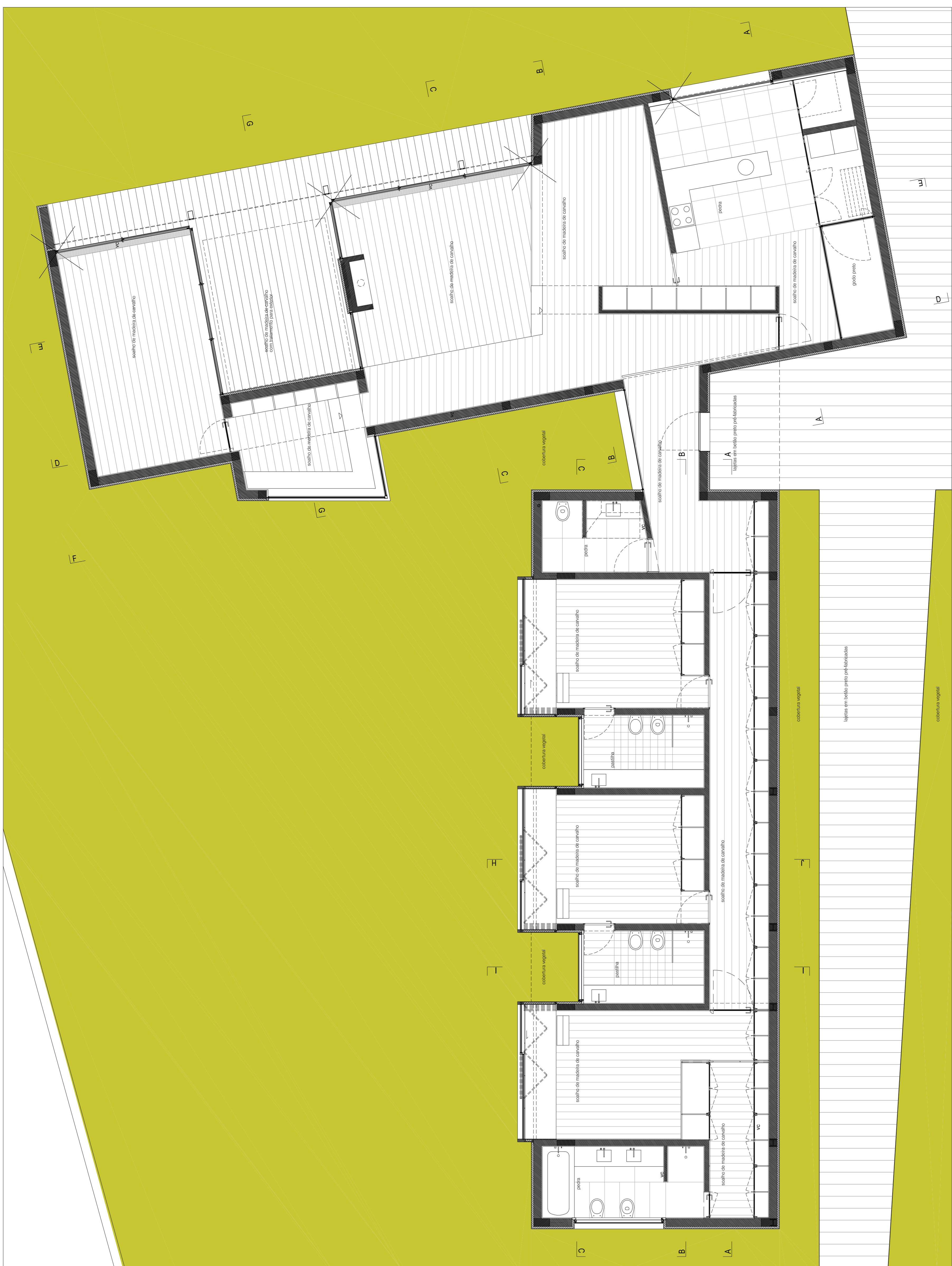
LEGENDA: 1.VESTIBULO 2.INSTALAÇÕES SANITÁRIAS (reservaço, b.cadêncas, c.suíte) 3.QUARTO (reservaço, b.cadêncas) 4.QUARTO DE VESTIR 5.CORREDOR (privado, b.socia) 6.CODINHA 7.LAVANDARIA 8.ARRUMOS SPATIO (alvarandaria, b.sala) 10.SALA DE JANTAR 11.SALA DE ESTAR 12.BIBLIOTECA 13.ESCRITÓRIO 14.MARANDA
