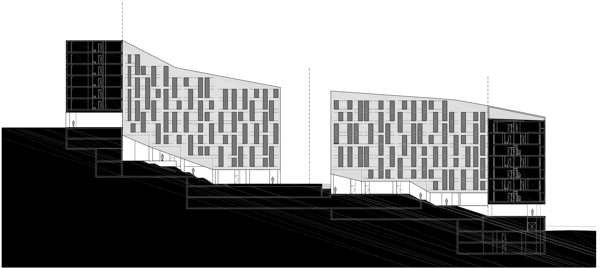
CORTE TRANSVERSAL / ALÇADO INTERIOR
